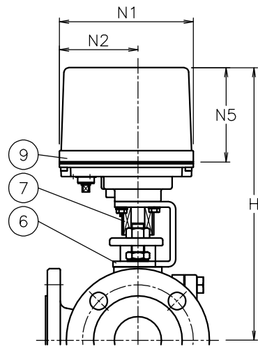
AE*L4*01DTT-050
