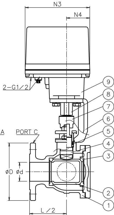
AE*L4*01DTT-025 AE*L4*01DTT-040
