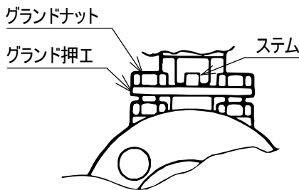
グランド締め付トルク [N・m]
